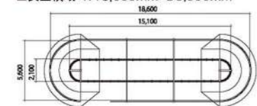
福島県福島市 蓬萊中央公園 BX1502 往復型: 滑走長約 33m
