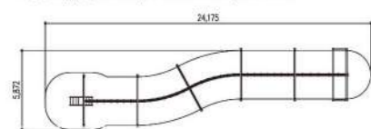
長崎県雲仙市 百花台公園 BX1506B ONE WAY 型: 滑走長約 24.5m
