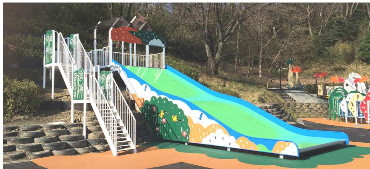
神奈川県横浜市 横浜こどもの国 幅 3m × 滑降長 9m
